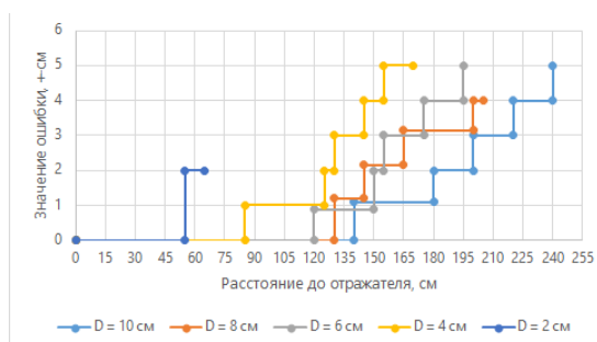
Рис.3. Зависимость погрешности в зависимости диаметра отражателя.
