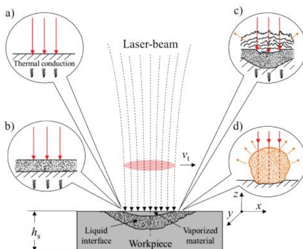
Рис.2– Схема облученного лазером материала: нагревание (thermal conduction – теплопроводность) (a), плавление (b), испарение и плавление (c) и образование плазмы (d)
