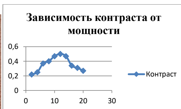
Рис.5 – график зависимости контраста изображения от мощности лазерного импульса
