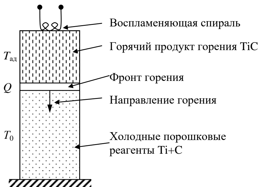
Рис. 1. Схема процесса получения карбида титана методом СВС
