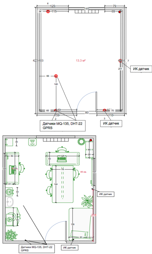
Рис 6. План кабинета с разметкой датчиков кабинета
