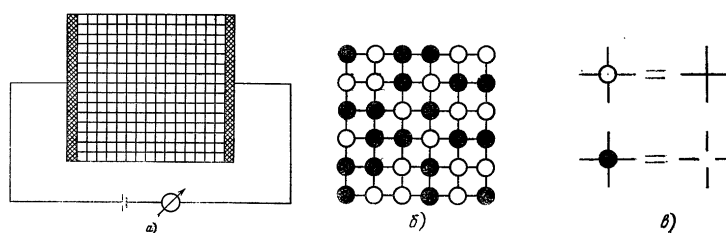
Рис. 1. Схема эксперимента из [1]. Число узлов уменьшено. а) Исходная сетка; б) кусок сетки с заблокированными узлами; в) черный узел – разрыв контакта между четырьмя проволоками, светлый узел сохраняет контакт
