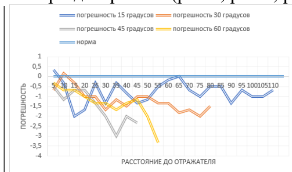
Рис.2. Зависимость погрешности вследствие изменения угла отражателя.
