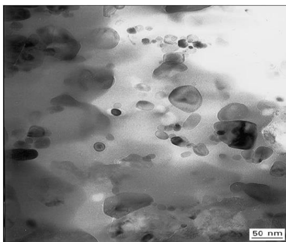
Рисунок 4. Структура толсто пленочного резистора в электронном микроскопе [9]
