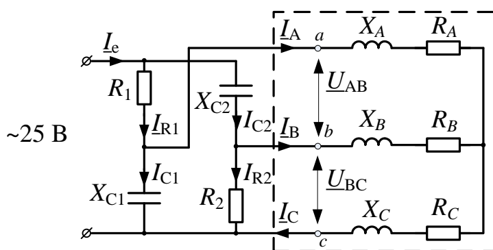
Рис. 1. Схема подключения трехфазного двигателя от одной фазы
