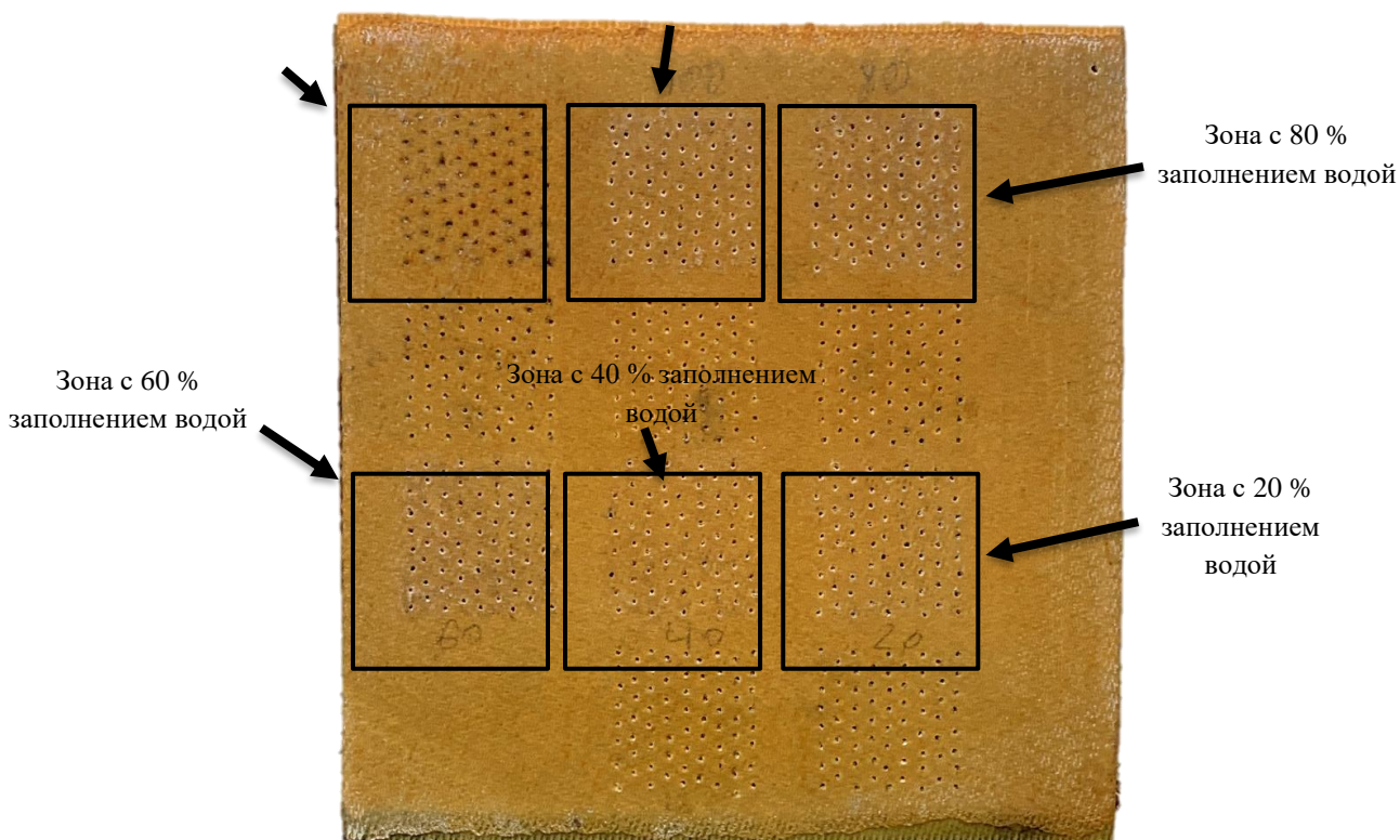
Рисунок 1– Тестовая сотовая панель (показаны отверстия в задней обшивке, через которые соты заполнялись водой и эпоксидным клеем)
