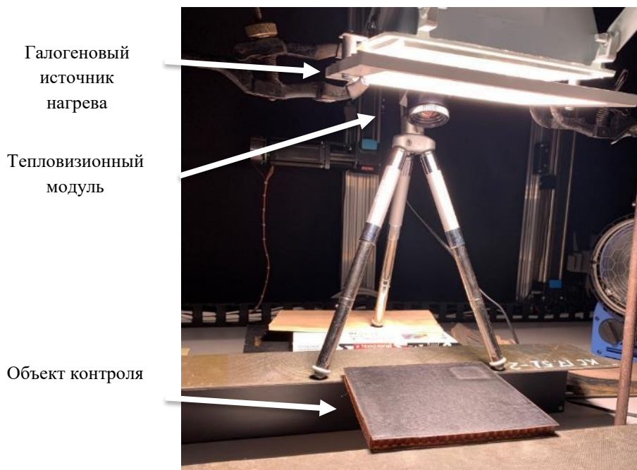
Рисунок 3 – Экспериментальная установка при контроле воды в сотах по схеме «снизу»
