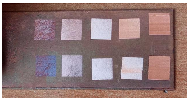
Рис.4 – лазерная гравировка меди при разной мощности излучения
