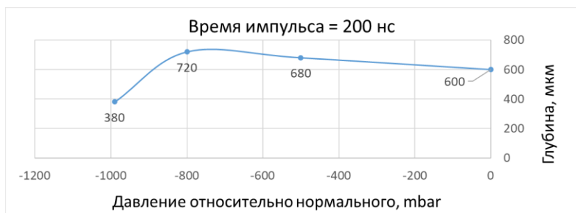
Рис. 3.1 – График зависимости глубины обработки от атмосферного давления (относительно н.у.) 200 нс
