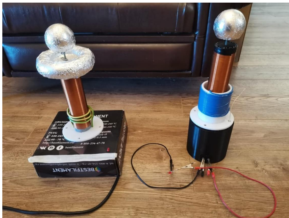
Рисунок 3. Трансформатор Теслы версии Качера Бровина.
