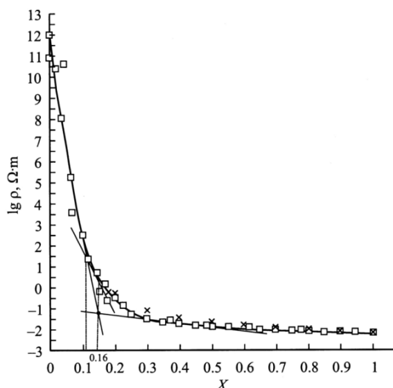
Рисунок 3. Зависимость удельного сопротивления парафин – графит от объемного содержания графита (в полулогарифмическом масштабе) □- эксперимент, × – теория [3]. Порог протекания составляет 16%
