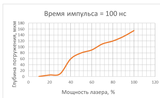
Рис. 2.2 – График зависимости глубины обработки от мощности лазера при времени импульса 100 нс
