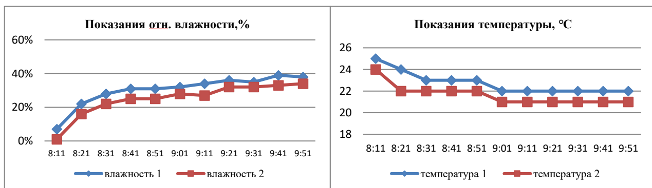
Рис 4. Показания датчиков, установленных в метре от увлажнителя воздуха
