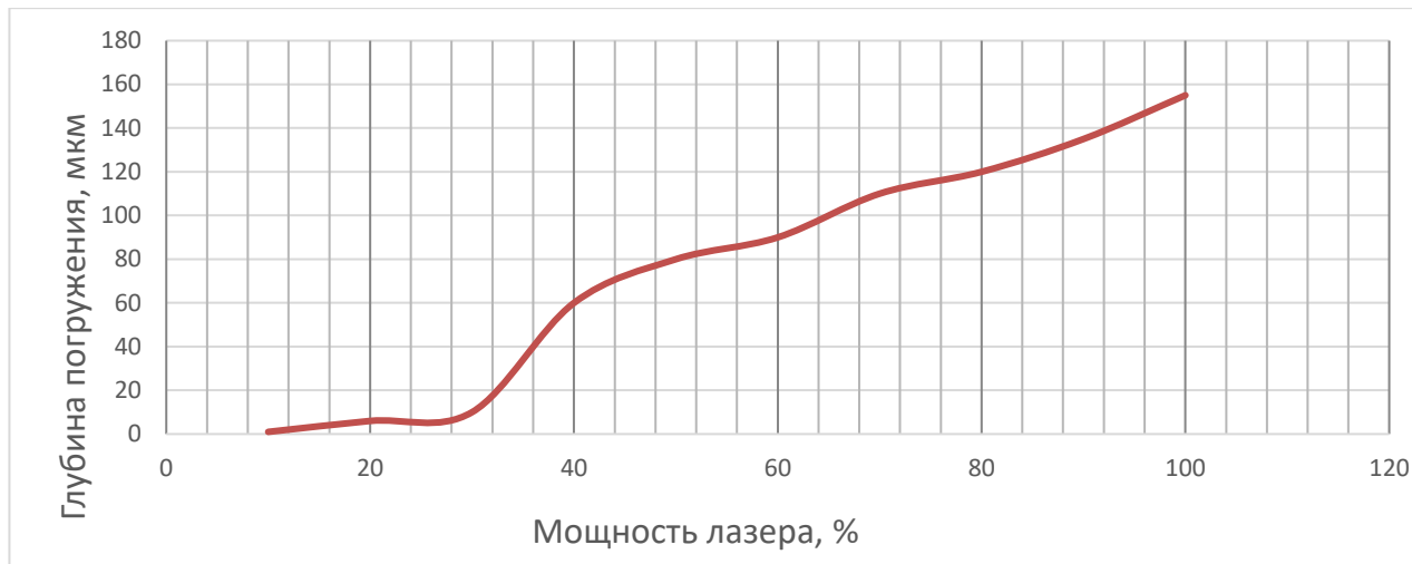
Диаграмма 2. Зависимость глубины от мощности при времени импульса 100нс.
