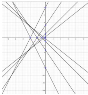
Рисунок 1. Прямые вида q = kp + b при фиксированном x \in [-2; 2]
