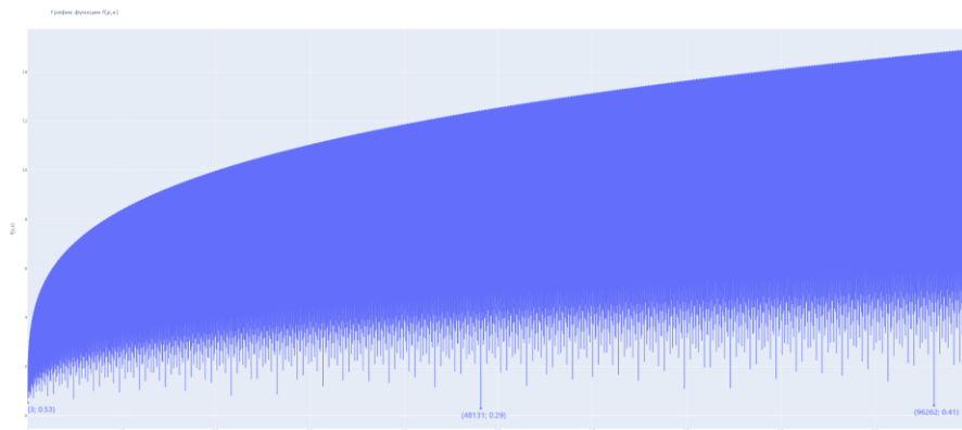
Рисунок 11. График функции f(\alpha; x) для \alpha = \rho на [1; 100\ 000] .
