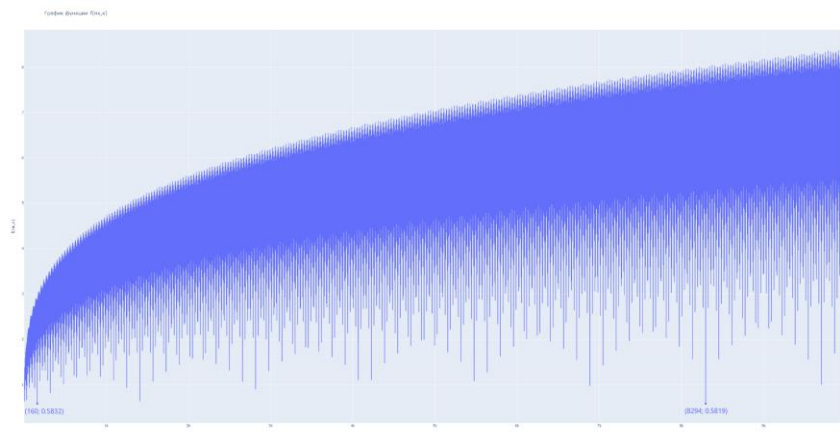
Рисунок 19. График функции f(\alpha; x) для \alpha = 1 пк на [1; 10\ 000] .
