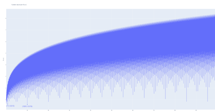
Рисунок 2. График функции f(\alpha; x) для \alpha = e на [1; 10\ 000] .
