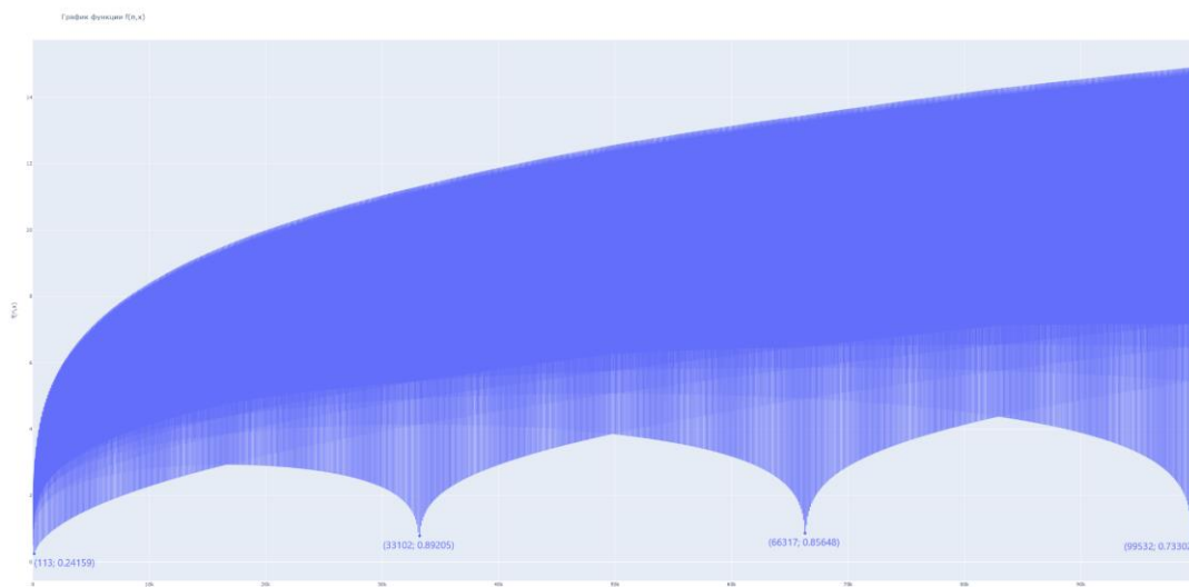
Рисунок 1. График функции f(\alpha; x) для иррациональных чисел на примере \alpha = \pi .
