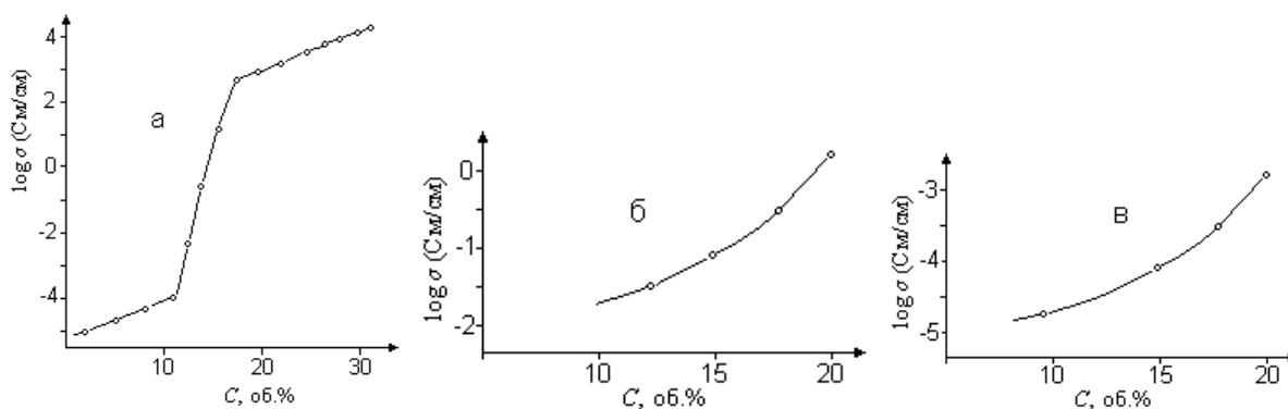
Рис.6. Зависимость проводимости легированного стекла от объемного содержания проводящей фазы для стекол: СЦНК-77-2 (а), С82-3 (б), С71-К (в)
