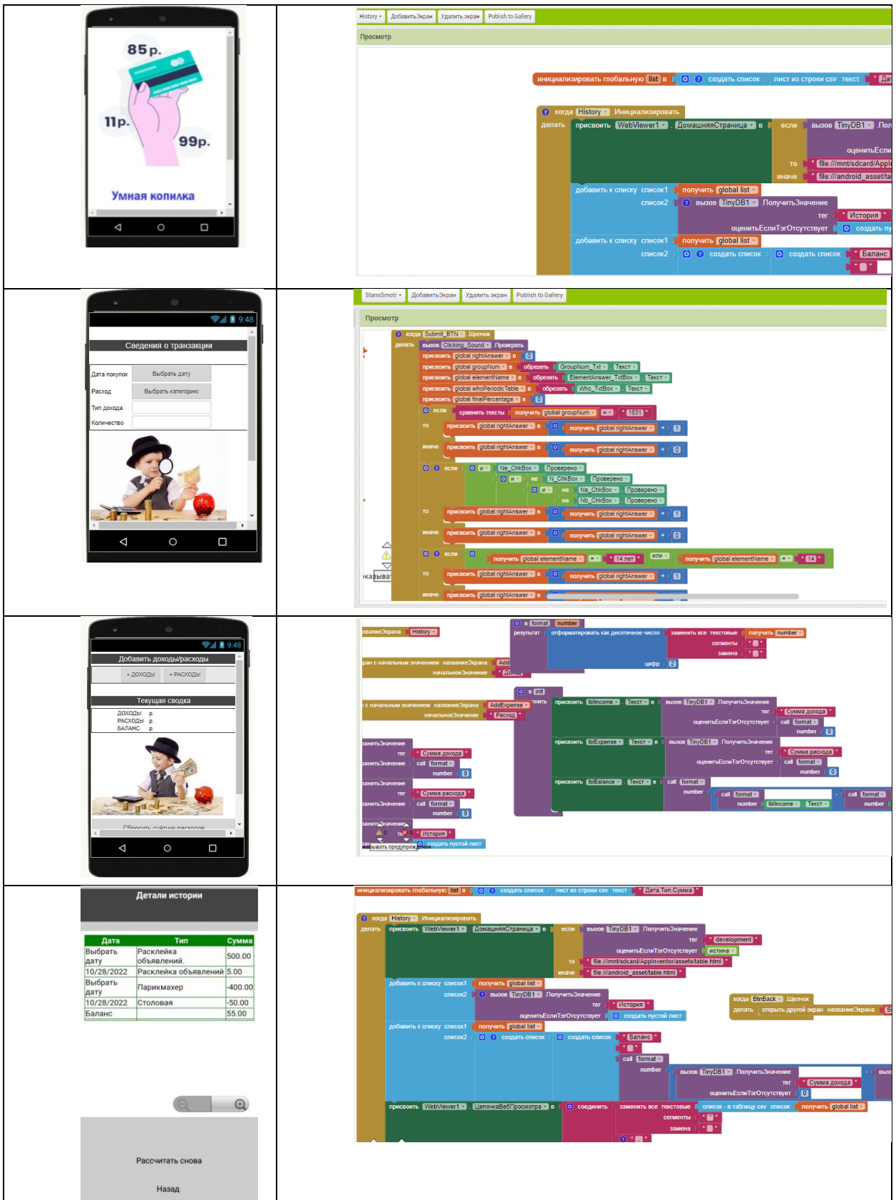
Рисунок 1. Интерфейс мобильного приложения в режиме «Дизайнер» и «Блоки»
