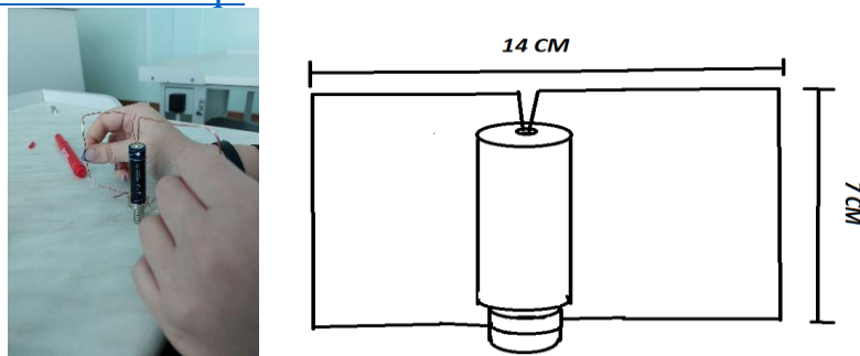
Рис 1. Фото и схема униполярного двигателя
