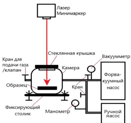
Рис 1. – Схема вакуумной камеры
