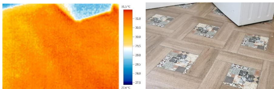
Рисунок 2 – Равномерность распределения теплового поля по поверхности.
