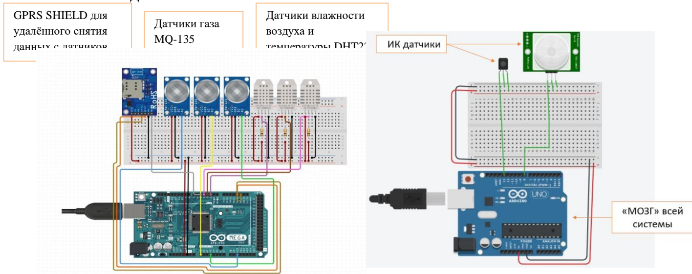
Рис. 1. Принципиальная схема подключения датчиков к Arduino
