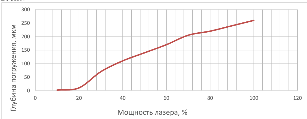
Диаграмма 1. Зависимость глубины от мощности при времени импульса 200нс.
