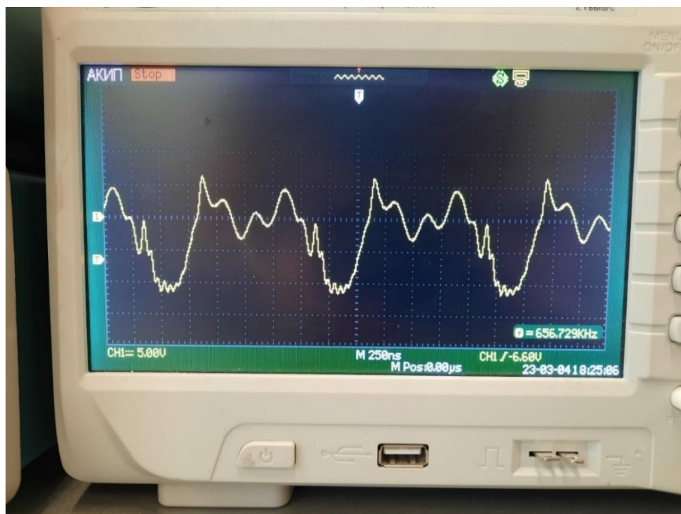
Рисунок 4. Синусоида выходного сигнала.
