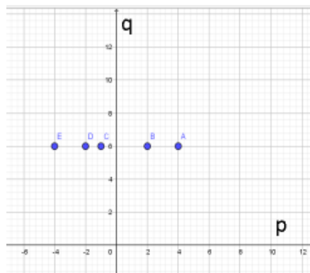
Рисунок 2. Точки в плоскости Orq
