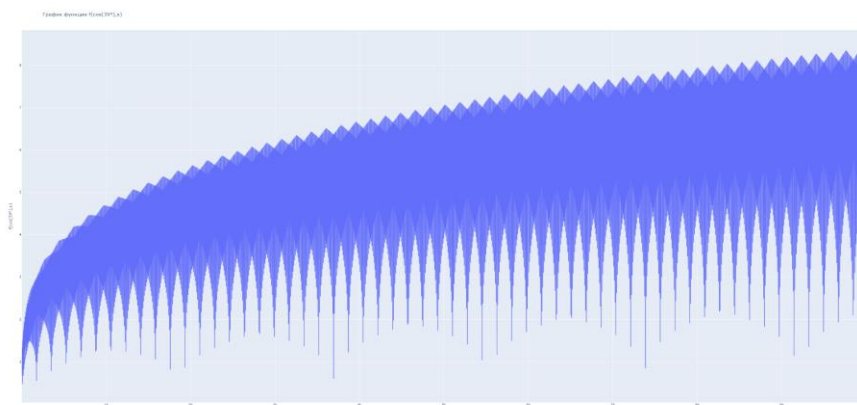
Рисунок 15. График функции f(\alpha; x) для \alpha = \cos(39^\circ) на [1; 10\ 000] .
