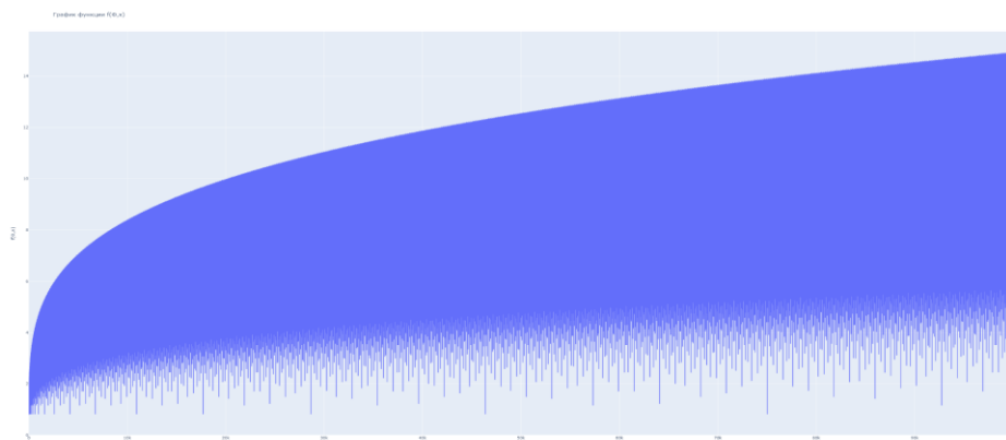
Рисунок 9. График функции f(a; x) для a = \Phi на [1; 100\ 000] .
