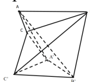
Рисунок 8. Невыпуклый многогранник, полученный с помощью поворота
