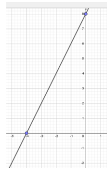
Рисунок 2. Прямая q = 2p + 8 на плоскости Орq.
