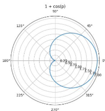
Рисунок 1. График кривой r = 1 + \cos \varphi в полярных координатах
