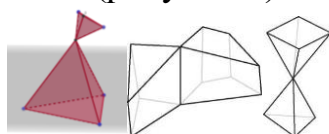
Рисунок 4. Две призмы с общей стороной и тетраэдры-близнецы
