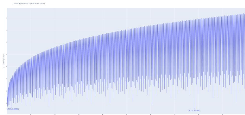
Рисунок 13. График функции f(\alpha; x) для \alpha = 5 + \sqrt[5]{\frac{467}{383}} на [1; 10\ 000] .
