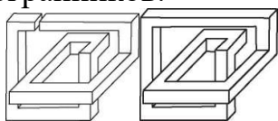
Рисунок 7. Два многогранника сложной формы
