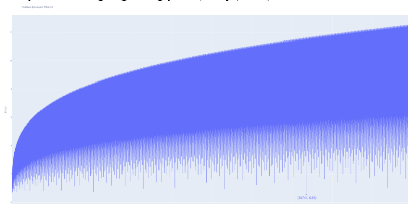
Рисунок 3. График функции f(\alpha; x) для \alpha = \ln 2 на [1; 50\ 000] .
