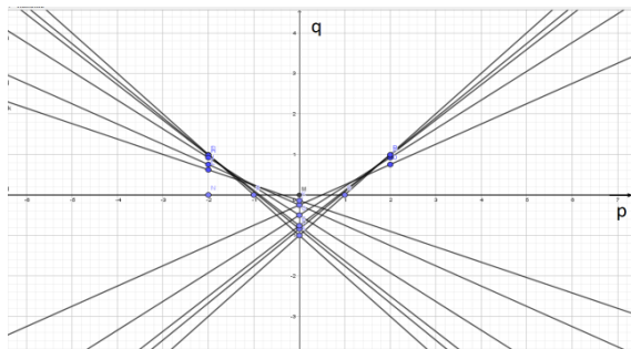
Рисунок 1. Построение прямых вида q = kp + b
