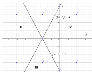
Рисунок 3. Прямые на плоскости Opq .
