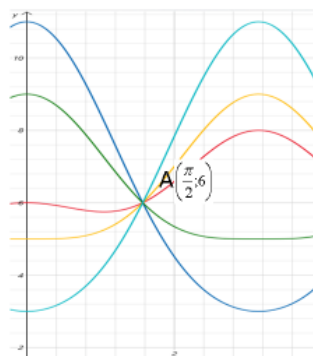
Рисунок 3. Графики функций в плоскости Oxy.
