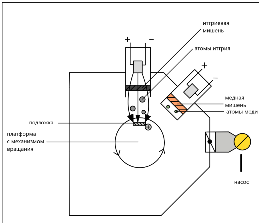
Приложение 2: схематичное представление процесса получения на подложке плёнки оксида иттрия
