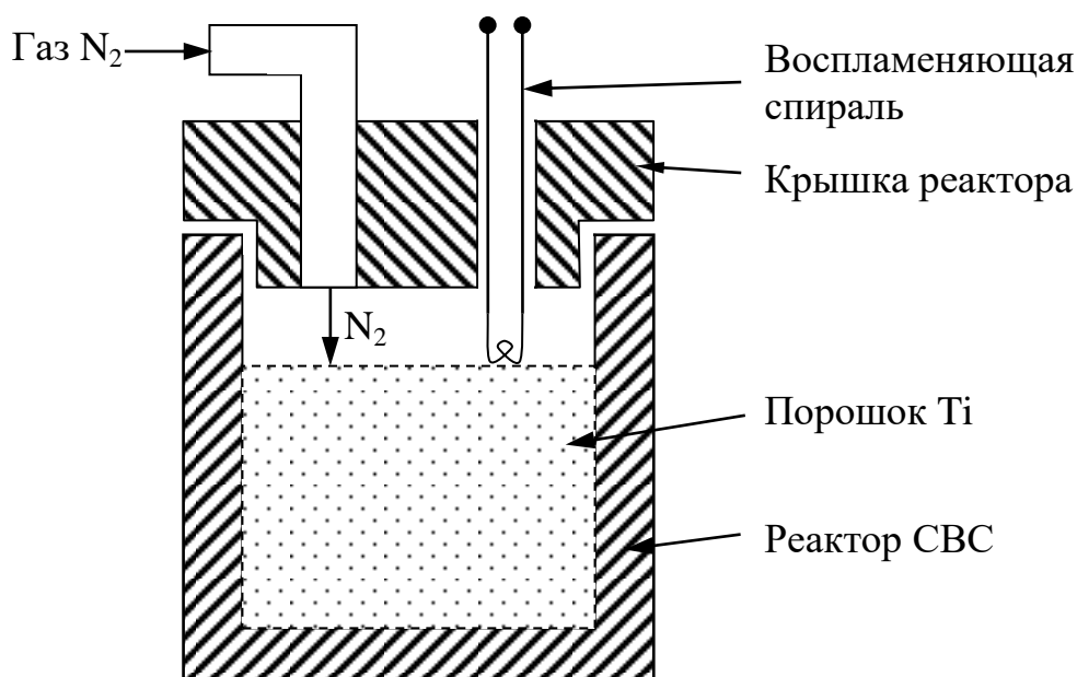
Рис. 2. Схема процесса получения нитрида титана методом СВС
