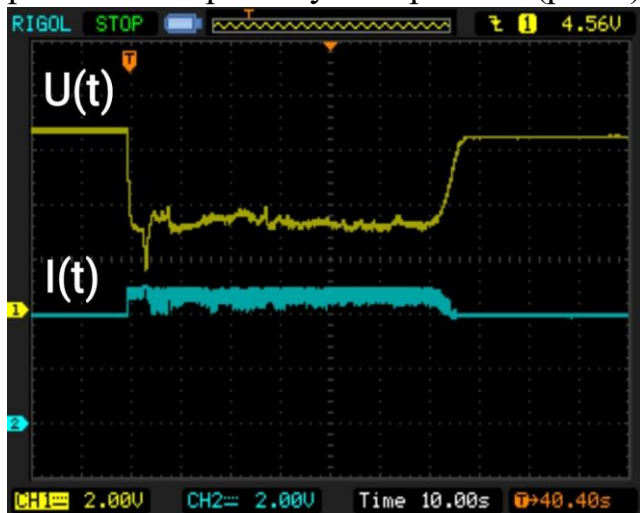
Рис. 1. Типичные характеристики процесса электродугового синтеза: U(t) - напряжение на источнике питания в процессе синтеза; I(t) - зарегистрированные значения тока в процессе синтеза.
